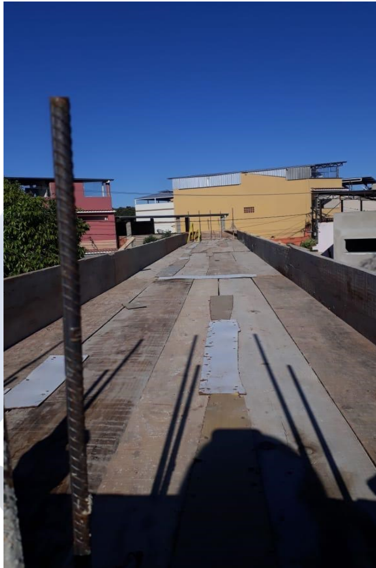
Foto 5: Montagem das formas da laje de sustentação do brise de estrutura metálica.
