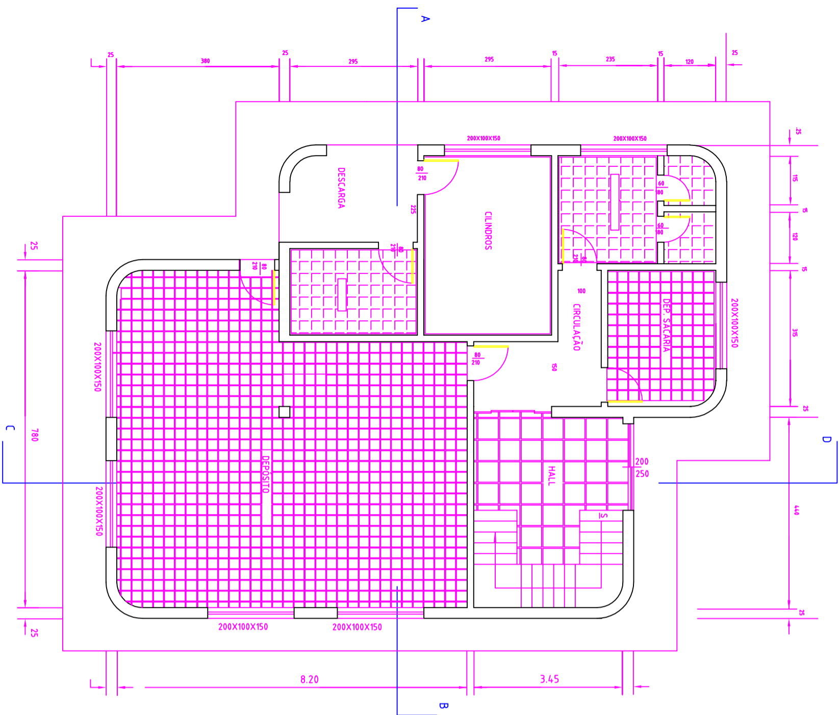
PLANTA BAIXA DO PAV. TÉRREO—ESC. 1:50
