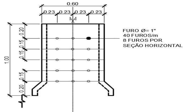
Esquema de furação do tubo de concreto perfurado - Classe PA-3/DN 600mm
