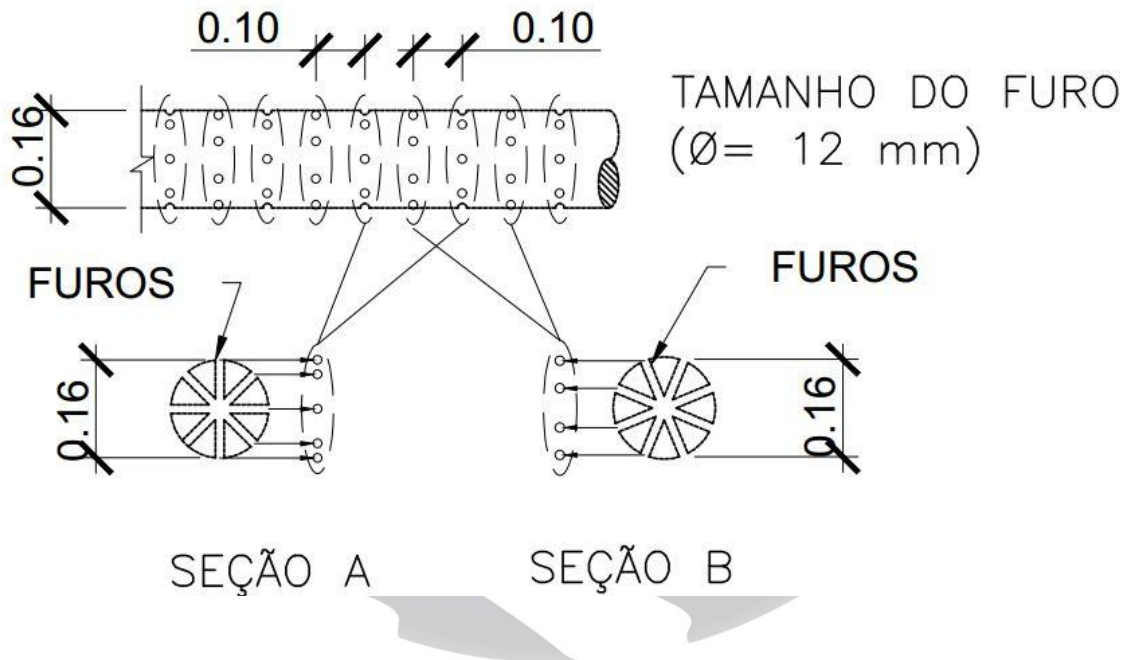
Esquema de furação do tubo de concreto perfurado - Classe PA-3/DN 600mm
